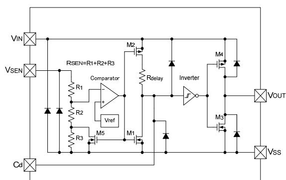
(2) XC6108CxxB
