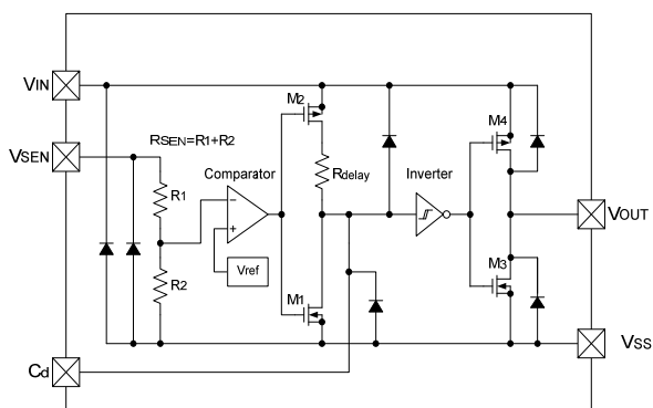
(3) XC6108NxxA
