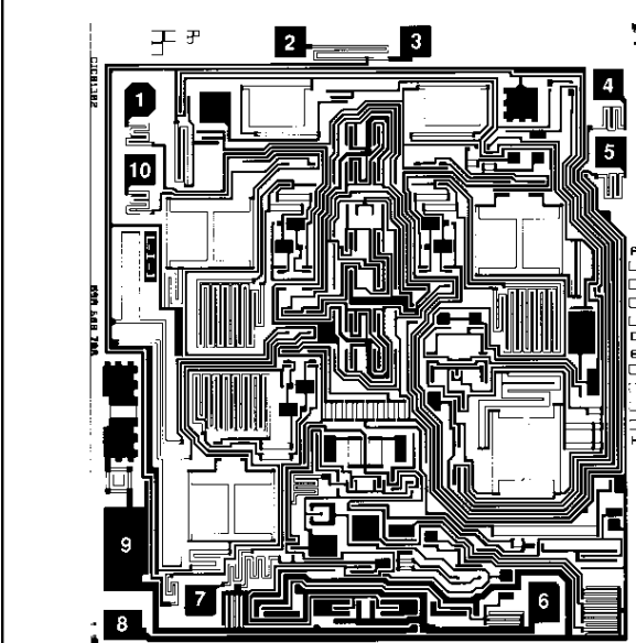
MPY100 DIE TOPOGRAPHY
