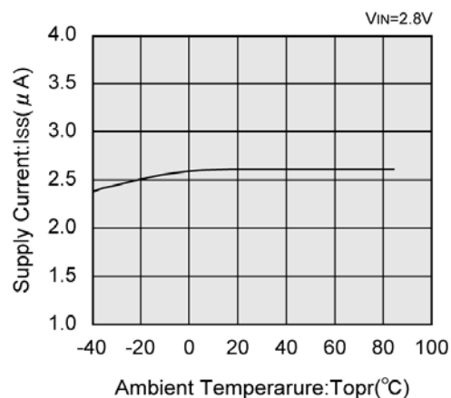
XC6201P182
