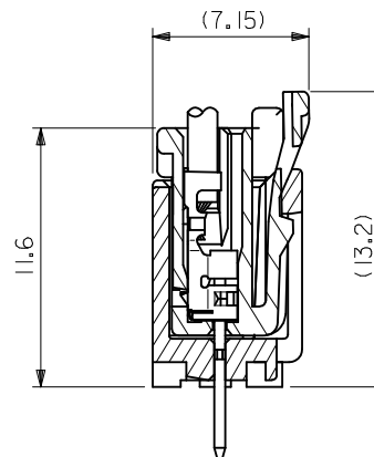
嵌合断面図
