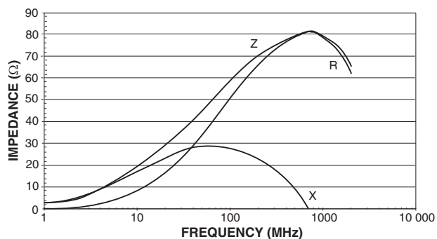
ILBB-0805 60 \Omega
