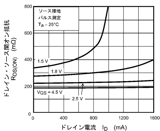
図 7.4 R_{DS(ON)} - I_D
