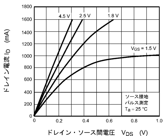
図 7.1 I_D - V_{DS}
