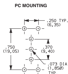
7101J1__BE2 SPDT
