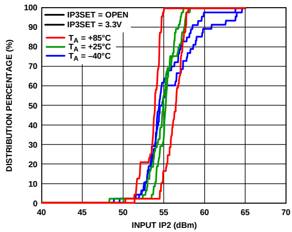
Figure 27. Input IP2
