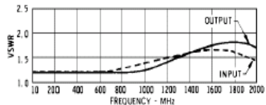
VSWR
