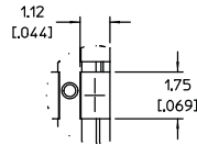
Detail A Scale 10:1 (4) PL.
