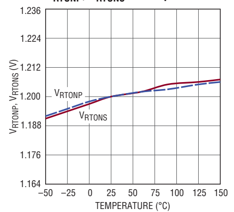
V_RT0NP, V_RT0NS vs Temperature
