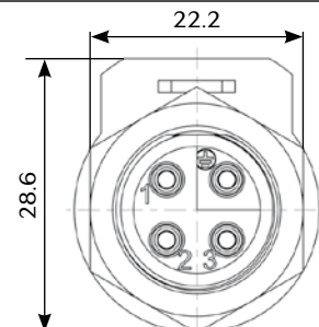
Wiring face
