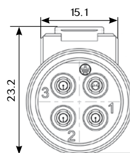
Wiring face
