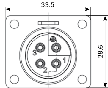
Wiring face
