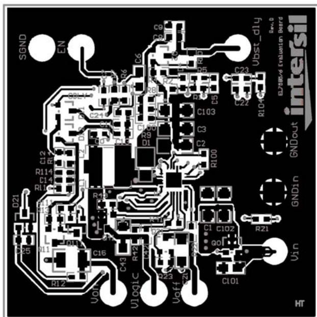
FIGURE 27. TOP LAYER
