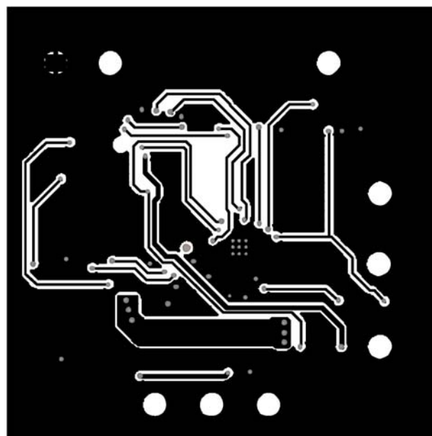
FIGURE 28. BOTTOM LAYER
