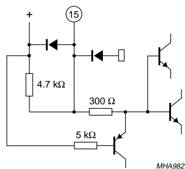
Fig.14 Pin 15; V CAP .
