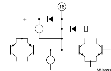
Fig.15 Pin 16; CAV.
