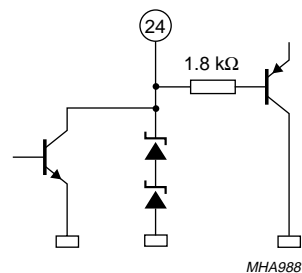
Fig.20 Pin 24; SDA.
