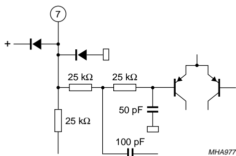
Fig.9 Pin 7; COMP.
