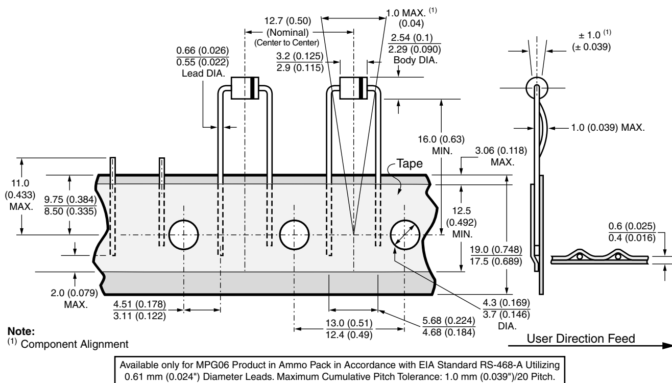
Fig. 4 - Pseudo Radial
