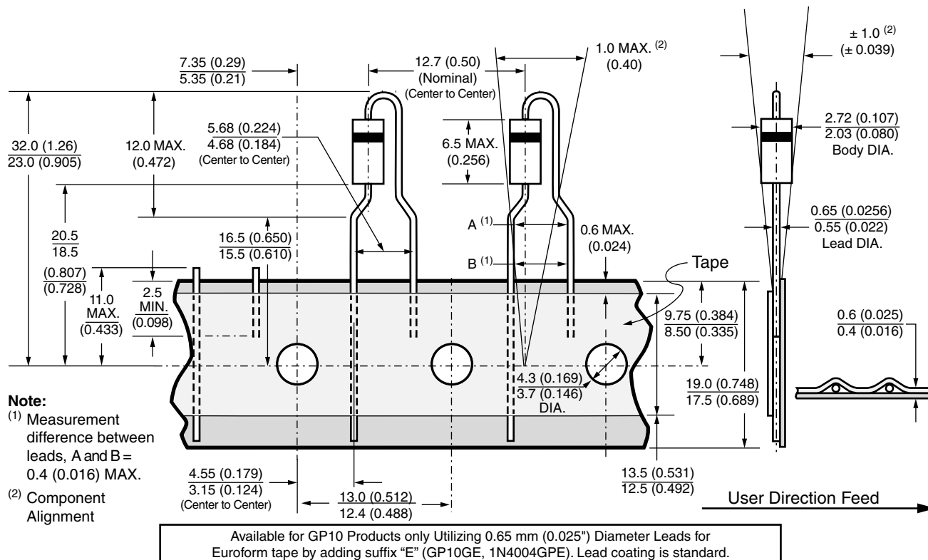
Fig. 3 - Euroform
