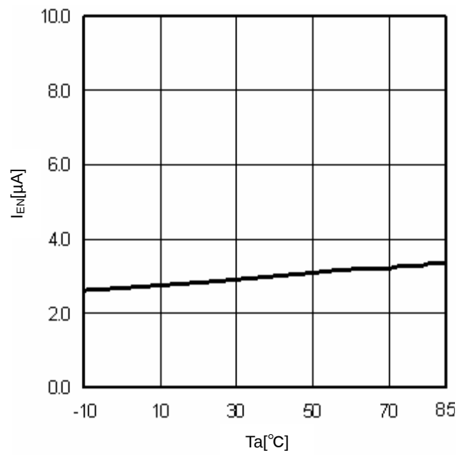
Fig.11 Ta-I EN
