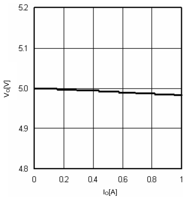
Fig.12 Io-V O
