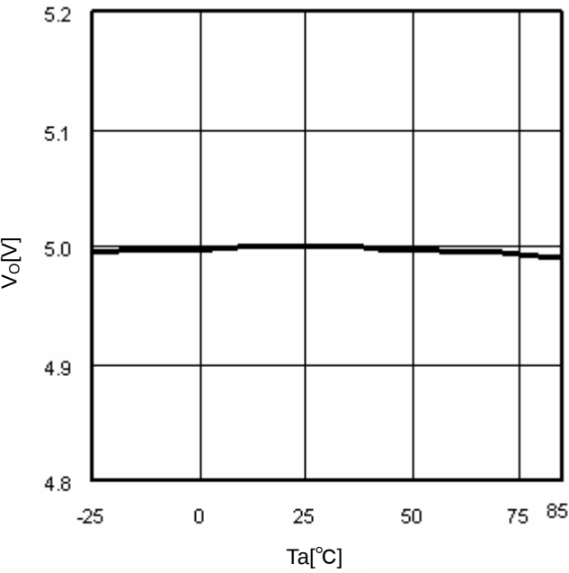
Fig.8 T_a-V_O ( I_o=0mA )
