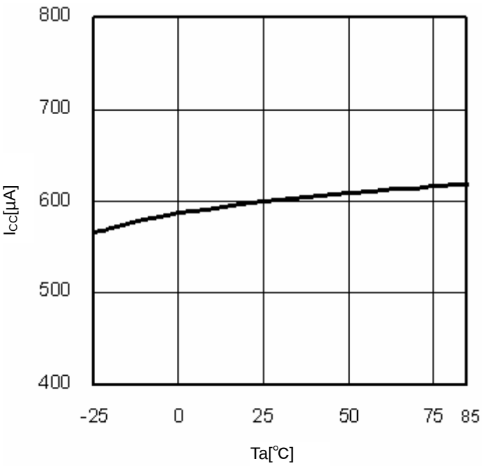
Fig.9 T_a-I_{cc}
