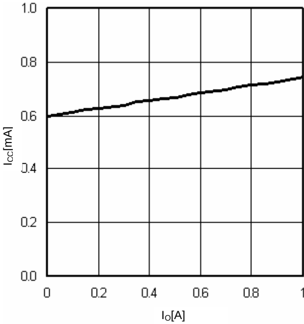
Fig.19 I_o - I_{cc}
