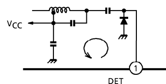
Fig.3 Rectifier Loop
