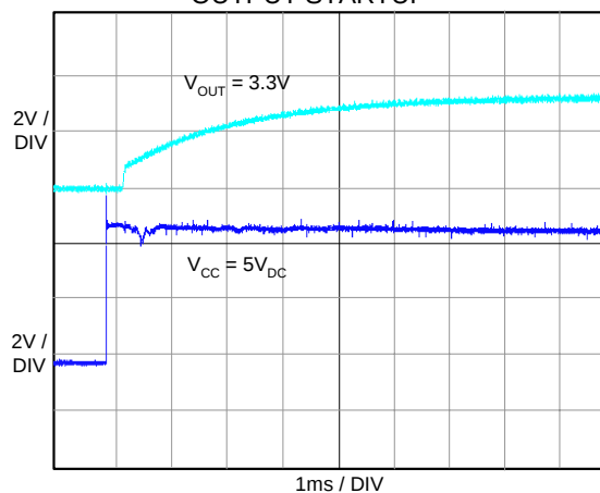
OUTPUT STARTUP
