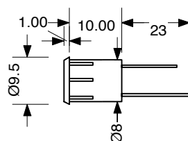
Body Dimensions
