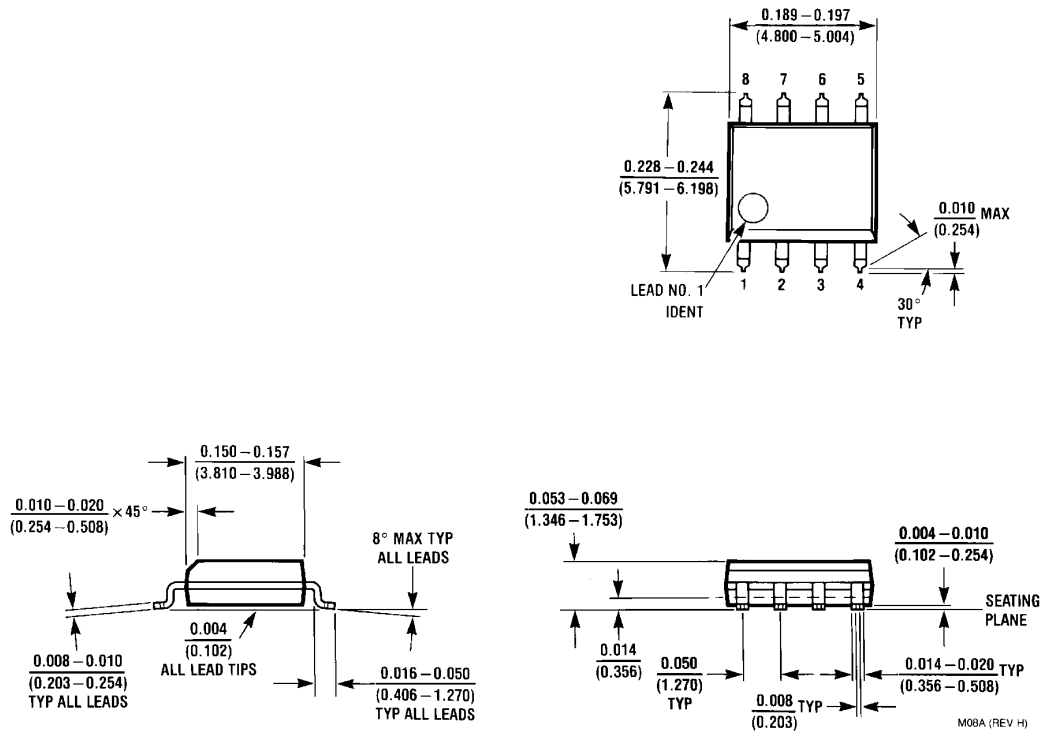
SO Package (M) Order Number LM334M, LM334MX, LM334SM or LM334SMX NS Package Number M08A
