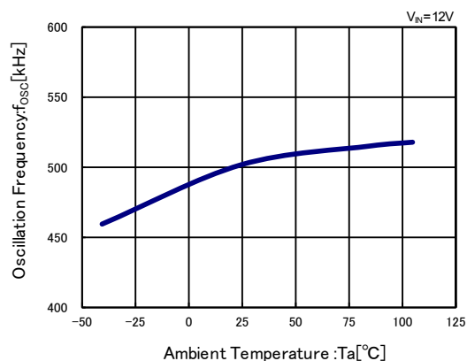
XC9263x755/XC9264x755 ( f_{osc}=500\text{kHz} )
