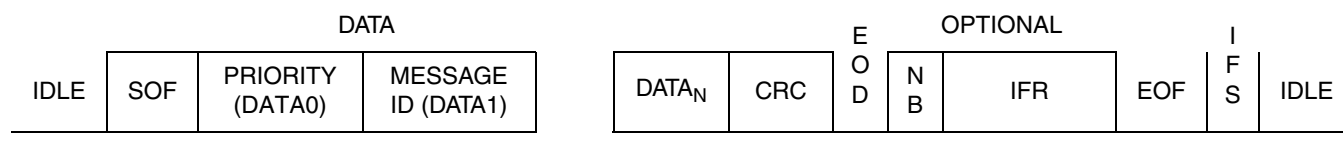
. J1850 Bus Message Format (VPW)
