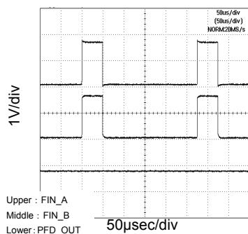
Fig.56 No Error Signal Output (VDD=3.3V, FIN_A = FIN_B)
