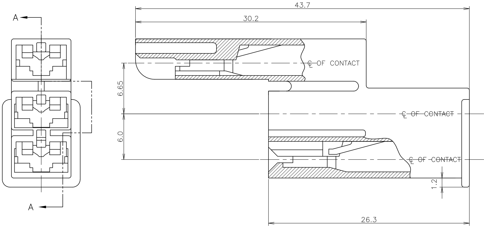
SECTION A-A
