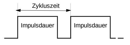
Bild 6-30 Impulsdauermodulation (PWM)
