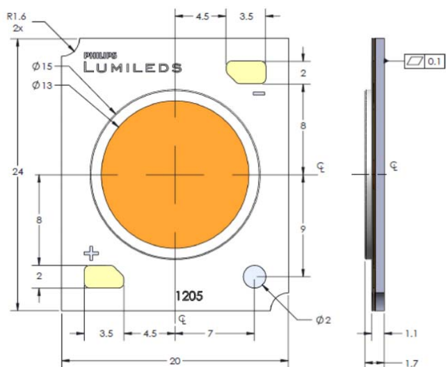
LUXEON CoB: LHCI – xxxx – I205
