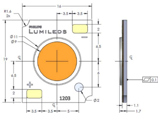
LUXEON CoB: LHCI – xxxx – I203
