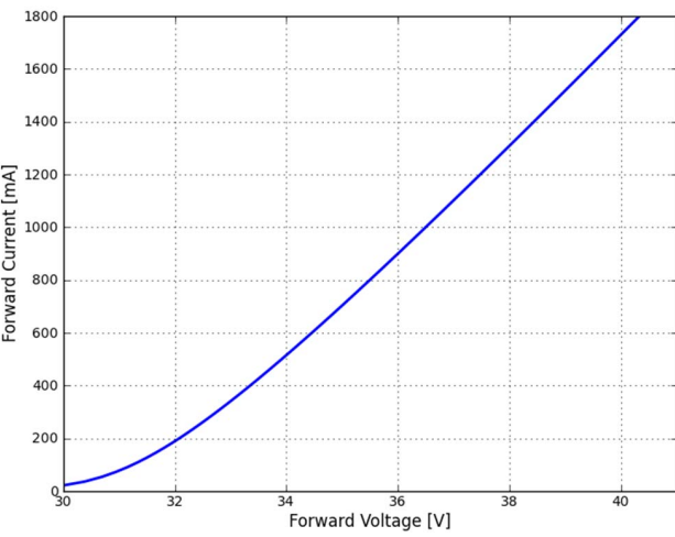
LUXEON CoB: LHCI – xxxx – I208
