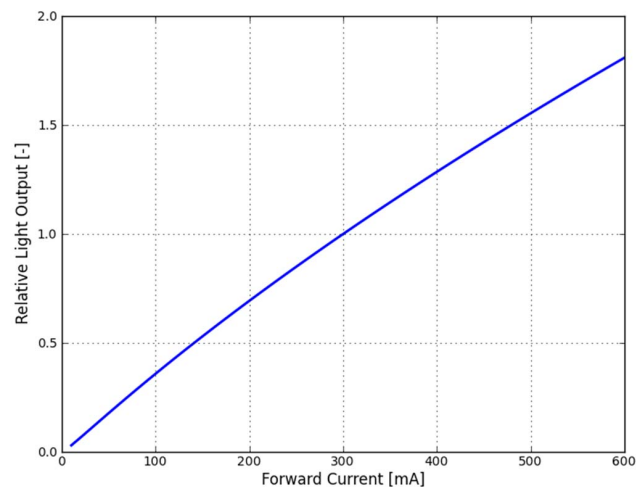
LUXEON CoB: LHCI – xxxx – I203
