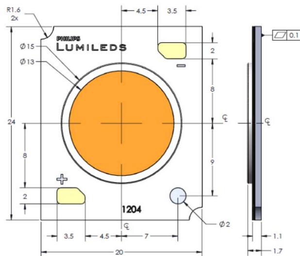
LUXEON CoB: LHCI – xxxx – I204
