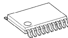
TSSOP20-P-0044-0.65
