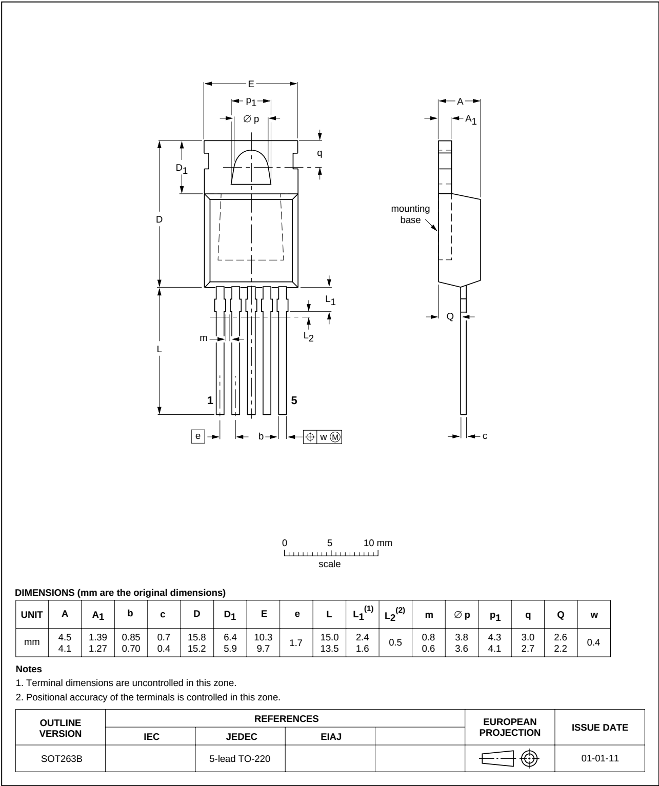
Fig 18. SOT263B.
