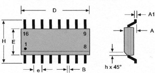
HMC1022—16-Pin SOIC
