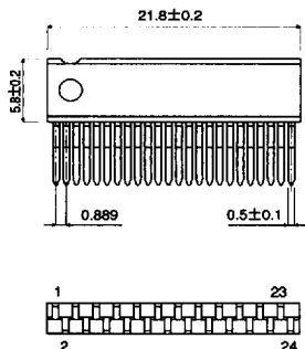
SZIP24
