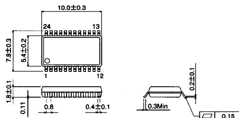
SSOP-A24
