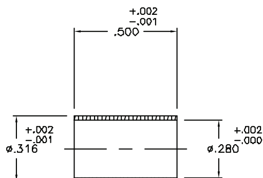
FERRULE
