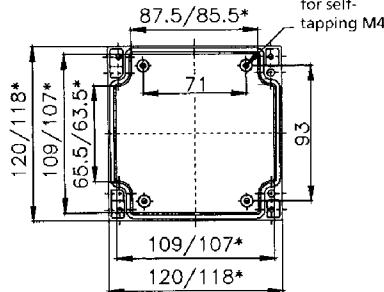
Lid
