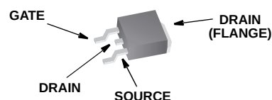
JEDEC TO-252AA
