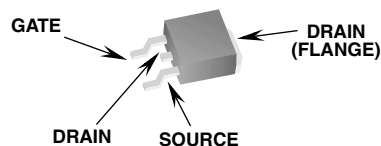
JEDEC TO-252AA
