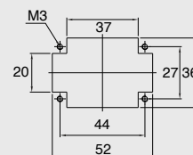
Montageausschnitt Panel cut-out
