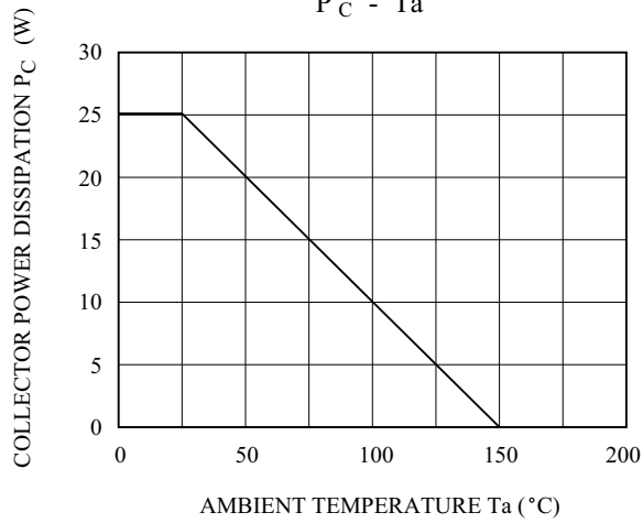
P_C - T_a
