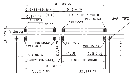
基板取付寸法
