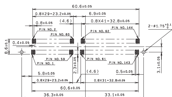
基板取付寸法
