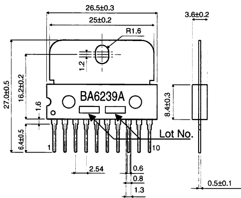
HSIP10 (Unit:mm)
