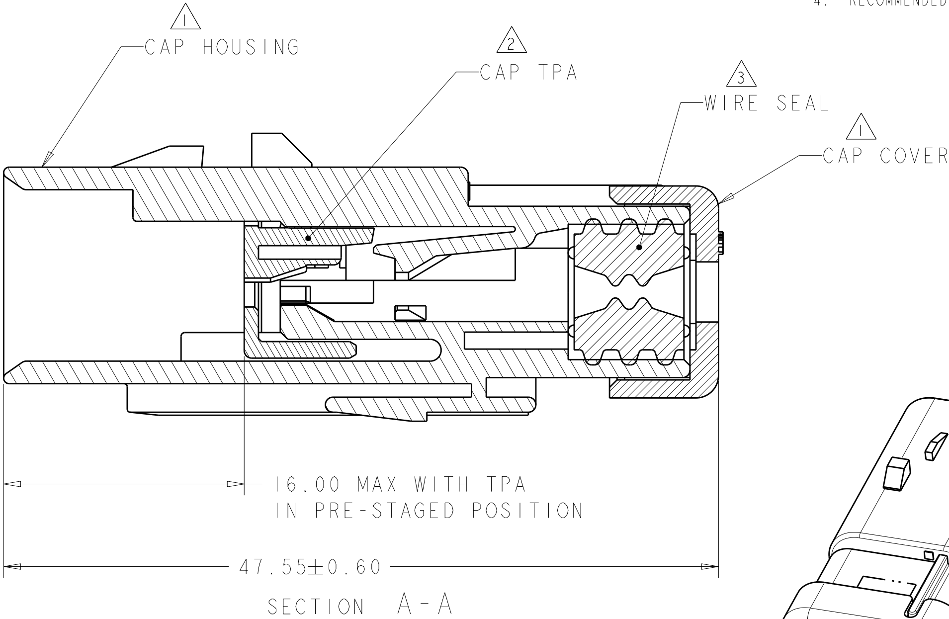
776535-4 SCALE 2:1 KEY D
