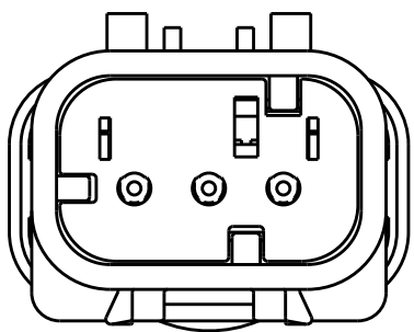
776535-3 SCALE 2:1 KEY C
