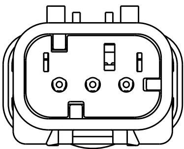
776535-2 SCALE 2:1 KEY B
