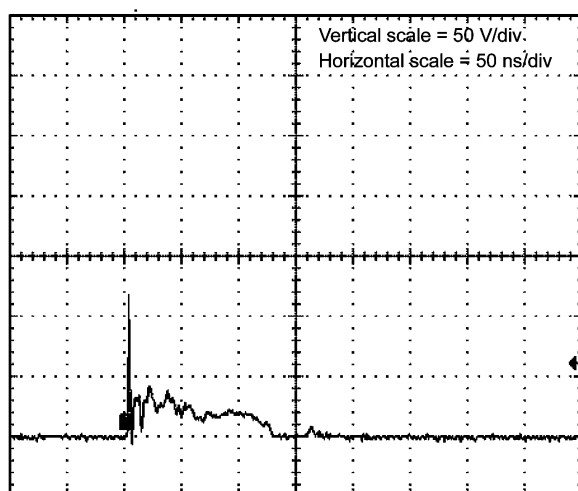
図 9.1 +8 kV
