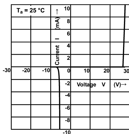
図 8.1 I - V
