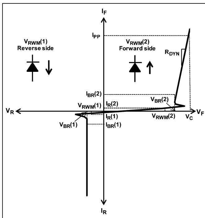
図 4.1 電氣的特性の定義
