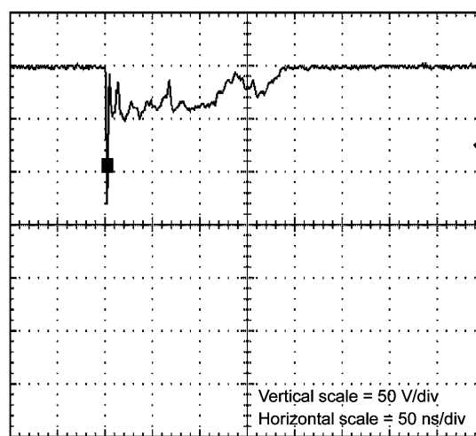
図 9.2 -8 kV
