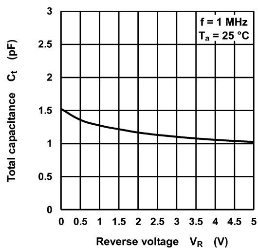
図 8.4 C_t - V_R
