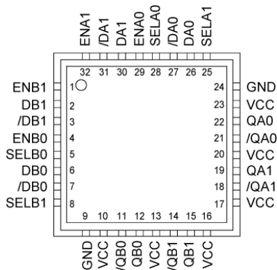
32-Pin EPAD-QFN
