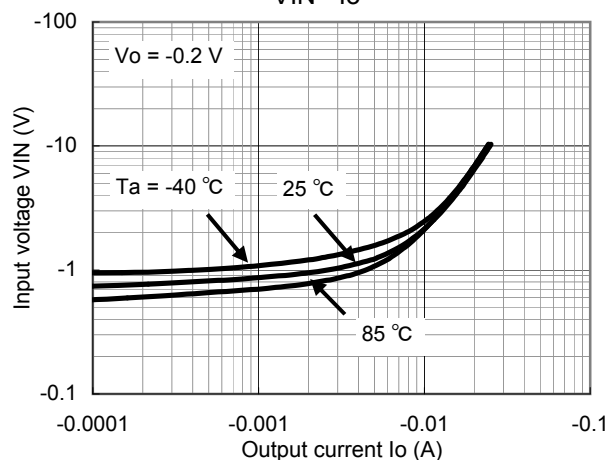
VIN - Io
