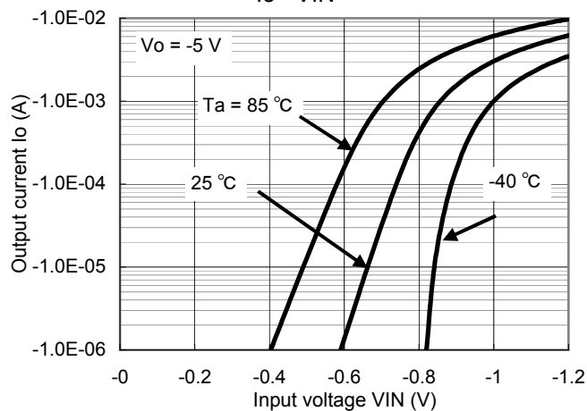
Io - VIN
