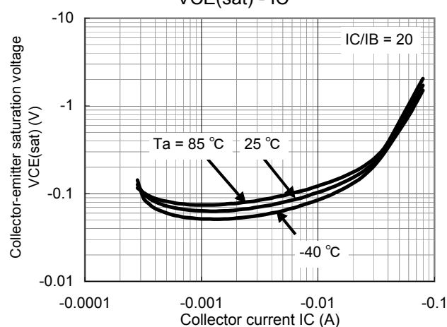
VCE(sat) - IC
