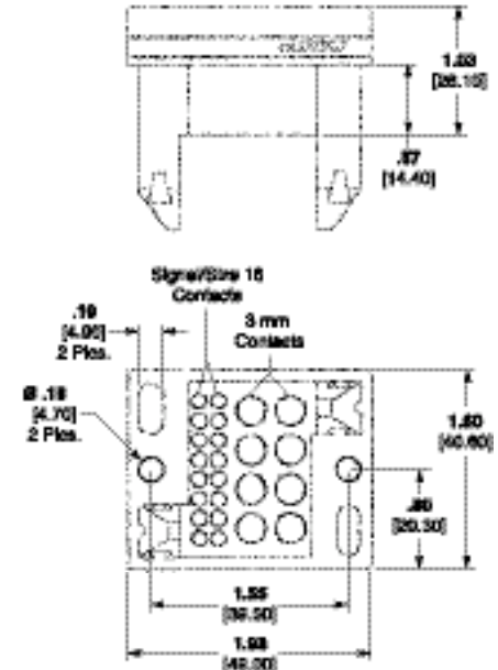
Plug 194298-1
