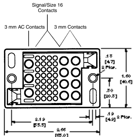
Plug 194242-1
