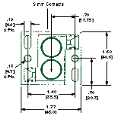
Plug 194282-1
