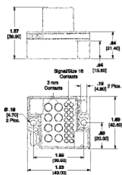
Receptacle 194299-1
