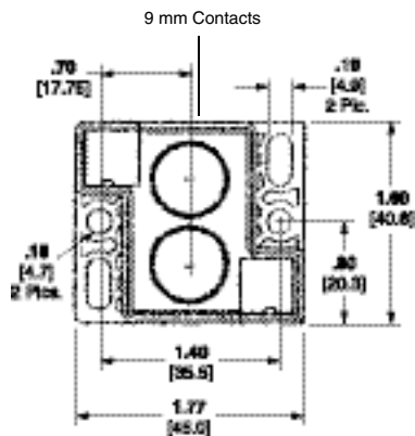
Receptacle 194283-1
