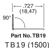
TB19 (1500)
