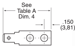
TB17 (1500)
