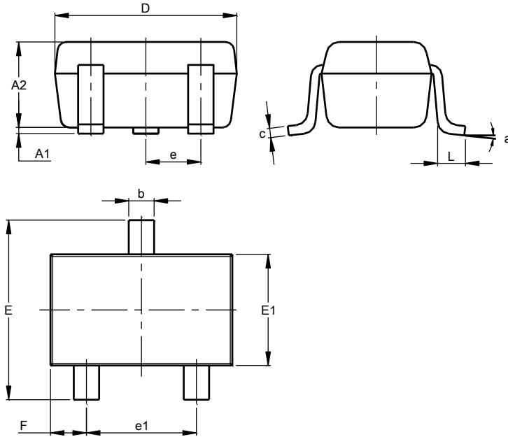
SOT323
