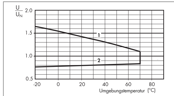
R 58 - AC-Spulen-Betriebsspannungsbereich
