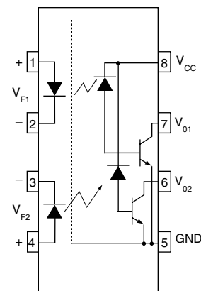
HCPL-2530/HCPL-2531
