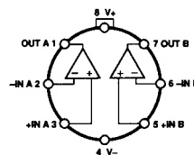
TO-99 (J-Suffix) OP-14
