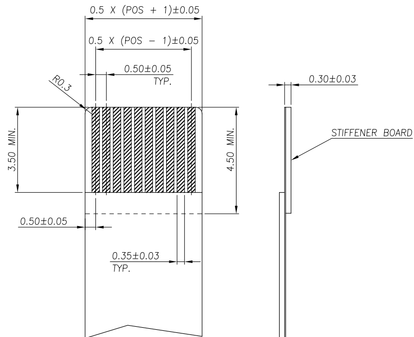
TOLERANCE \pm 0.05
