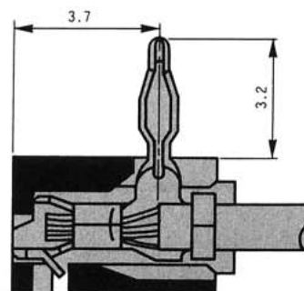
水平型装着断面 Right Angle Type Cross Cut Section
